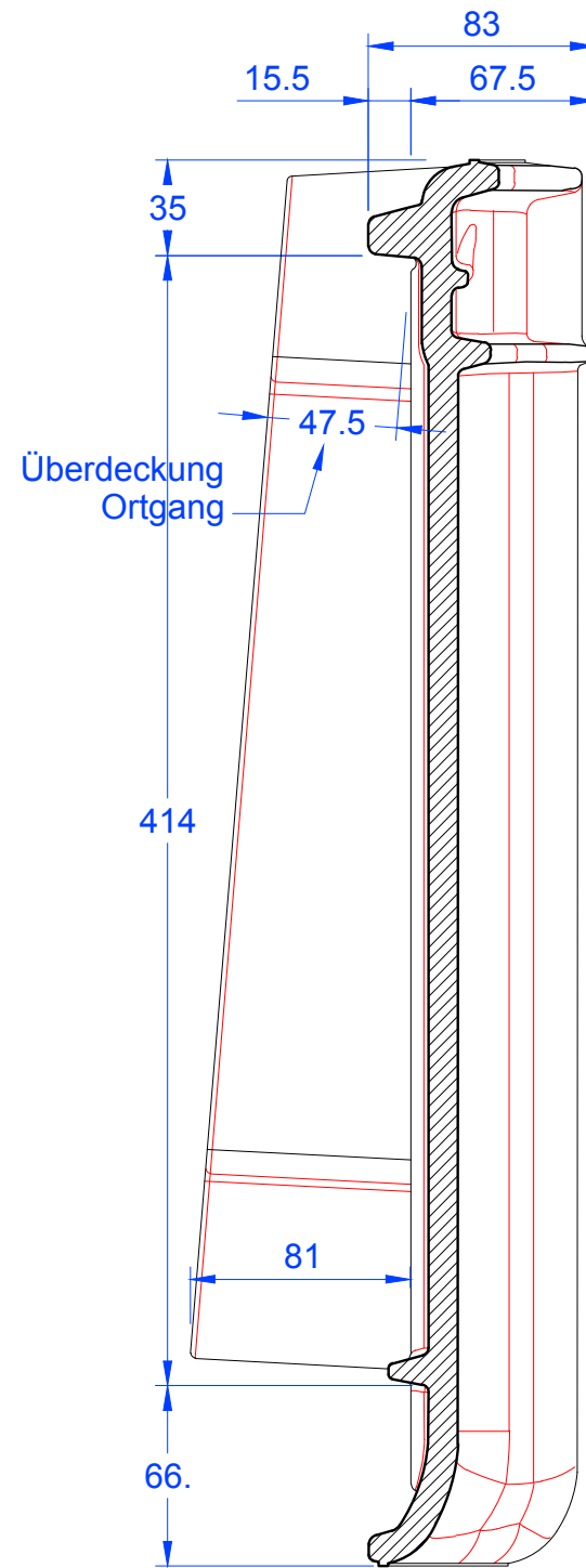
Schnitt B-B
